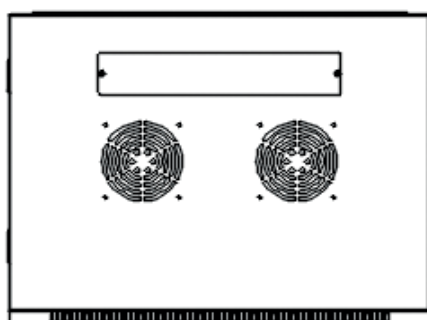
VISTA DALL'ALTO
