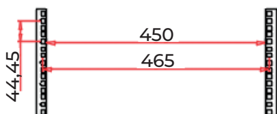
DIMENSIONI STANDARD RACK 19''
