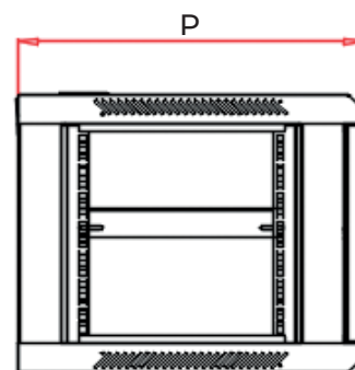
VISTA LATERALE SENZA PANNELLO
