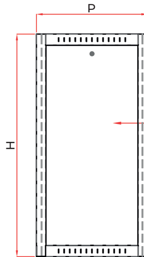
Vista laterale
