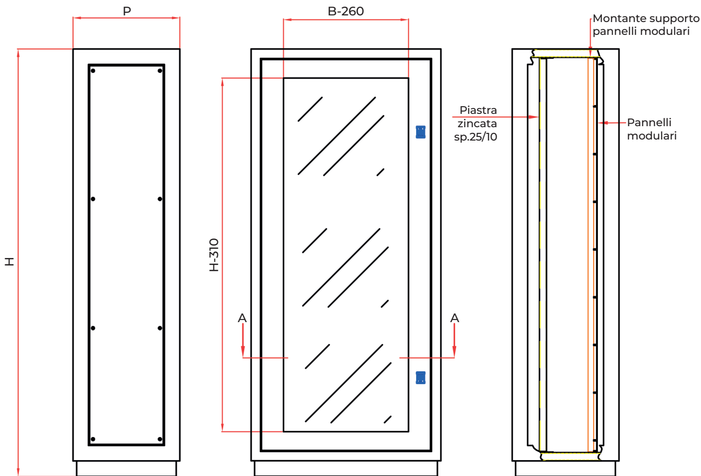
SEZ. A-A
