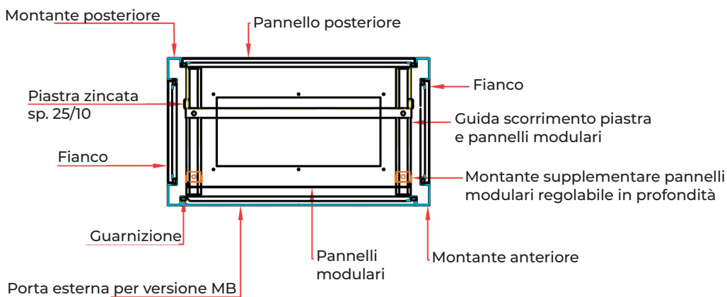
SEZ. A-A
