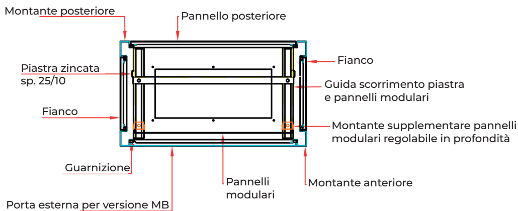
SEZ. A-A
